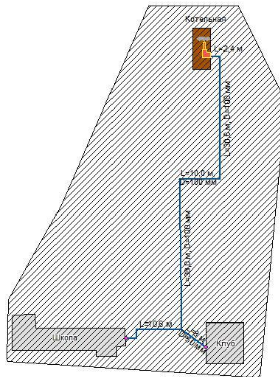
Рисунок 4 – Зона действия котельной №32 (с. Николай-Поль, Рабочий пер. №3)
