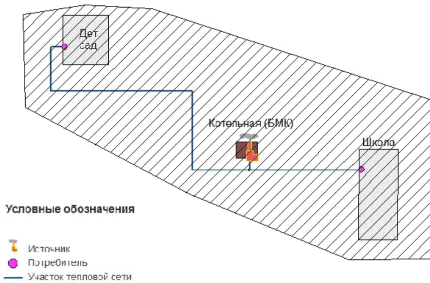
Рисунок 3 – Зона действия Блочно-модульной котельной школы и детского сада (д. Пучково, ул. Чкалова, 38);
