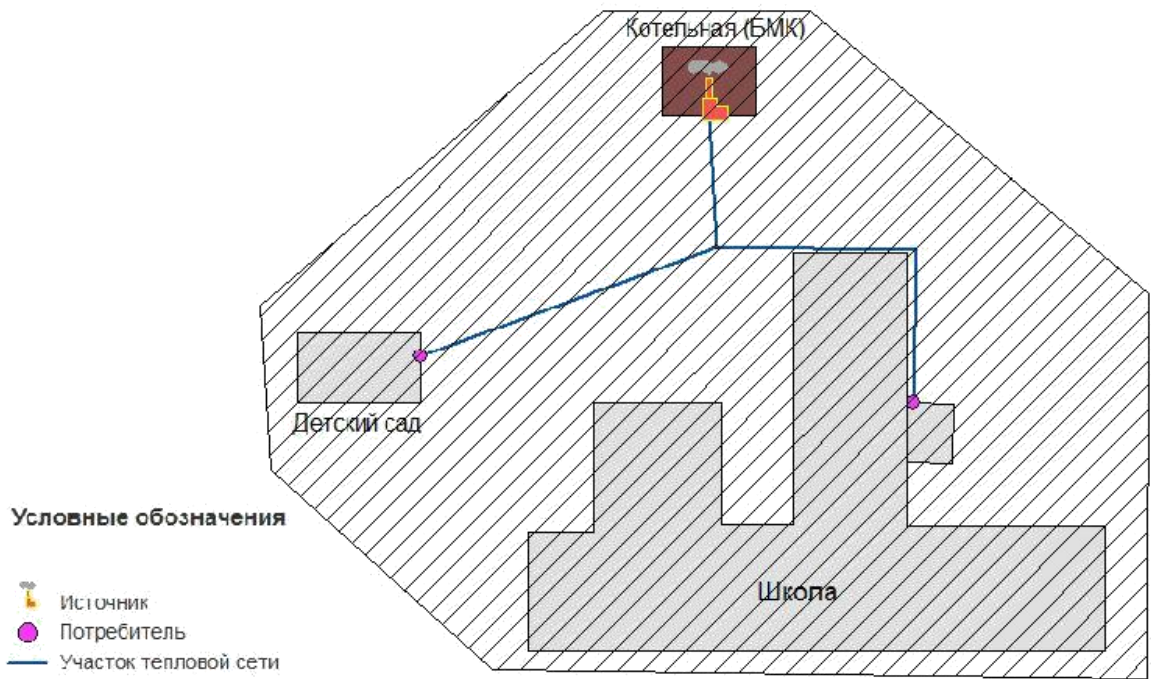
Рисунок 1 – Зона действия Блочно-модульной котельной школы и детского сада с. Маргелану
