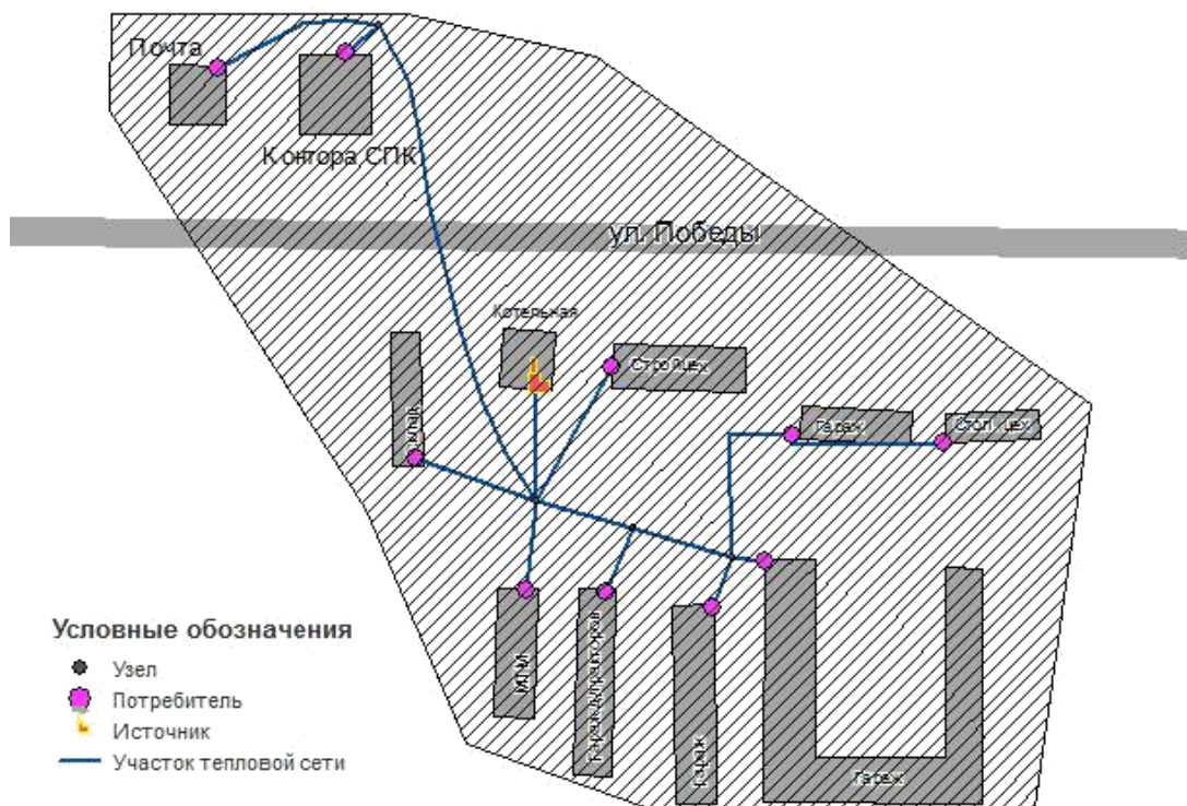
Рис. 2. Зона действия котельной СПК «Украинское»
