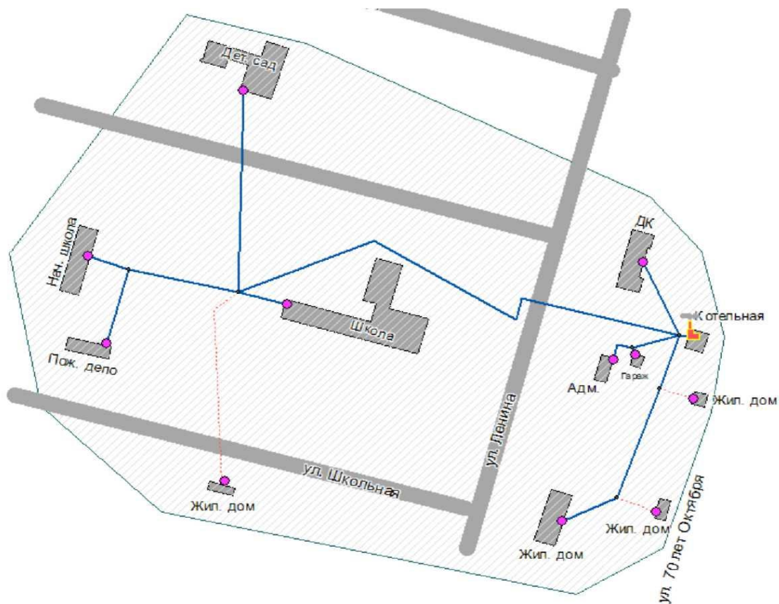
Рис. 1. Зона действия котельной №№31 (с. Украинка, ул. Школьная №4)
