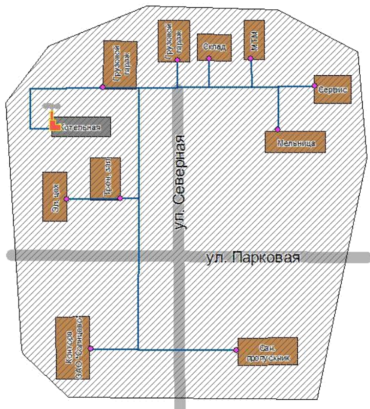
Рис. 2. Зона действия котельной ЗАО «Солнцево» (с. Солнцевка)
