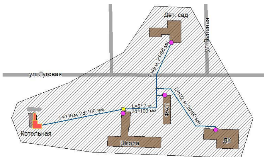
Рис. 1. Зона действия Котельной №24 (с. Первотаровка, ул. Центральная №26)
