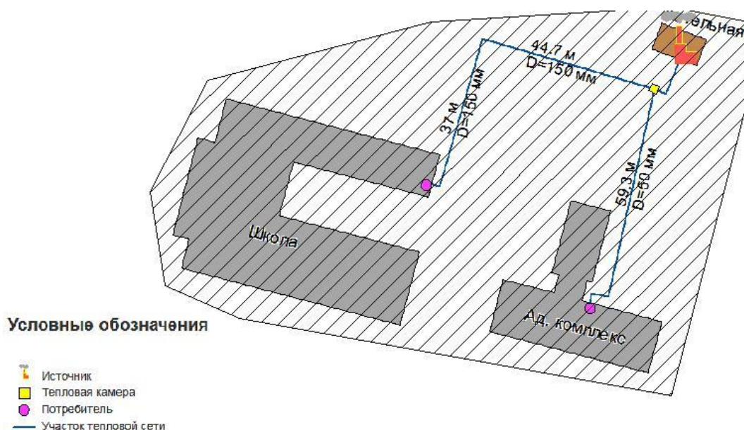
Рис. 1. Зона действия Котельной №28 (с. Новорождественка, ул. Школьная №3)
